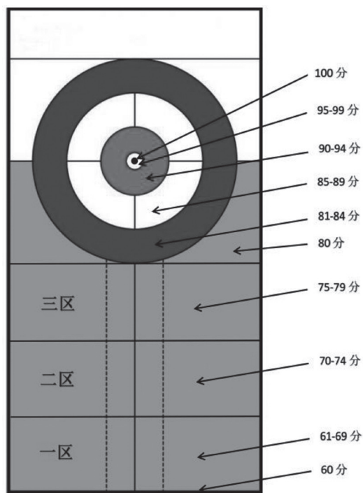
图 5-1 分值示意图
